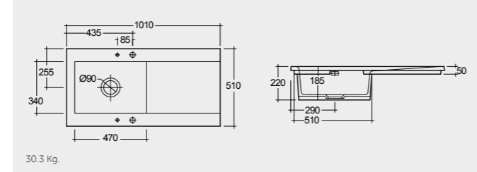
Right: OC201RHSLAWHA External overflow optional AWH Left: OC201LHSLAWHA No tap hole: OC201NTSLAWHA
