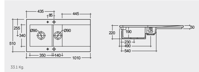
Right: OC200RHSLAWHA External overflow optional AWH Left: OC200LHSLAWHA No tap hole: OC200NTSLAWHA
